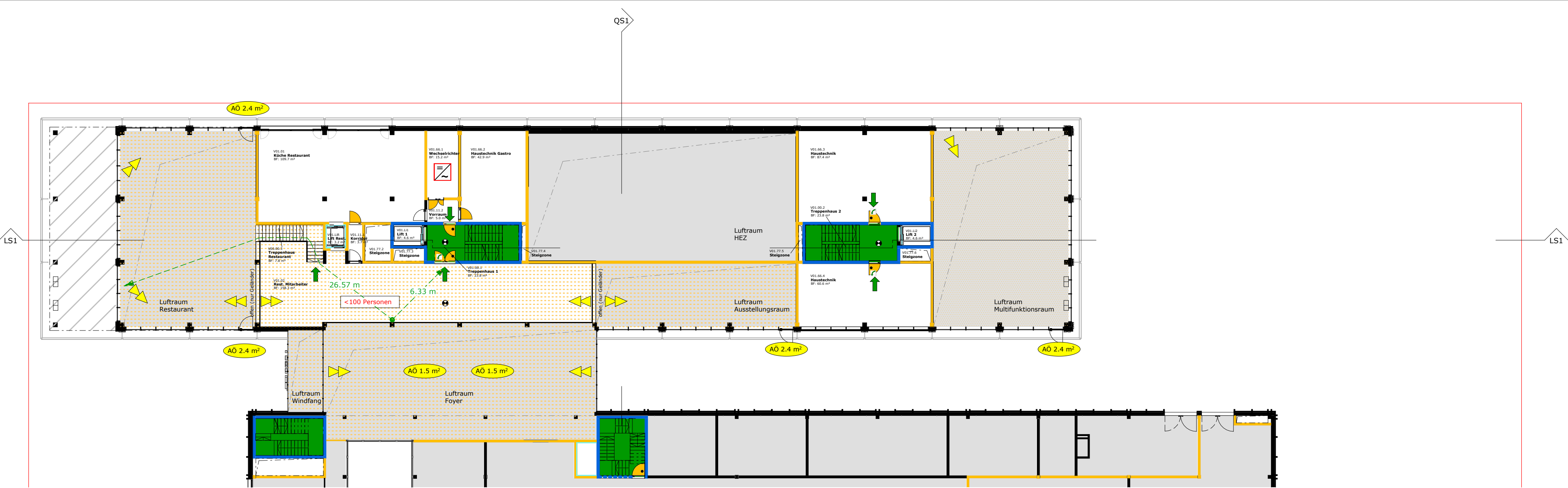
Grundriss V01
