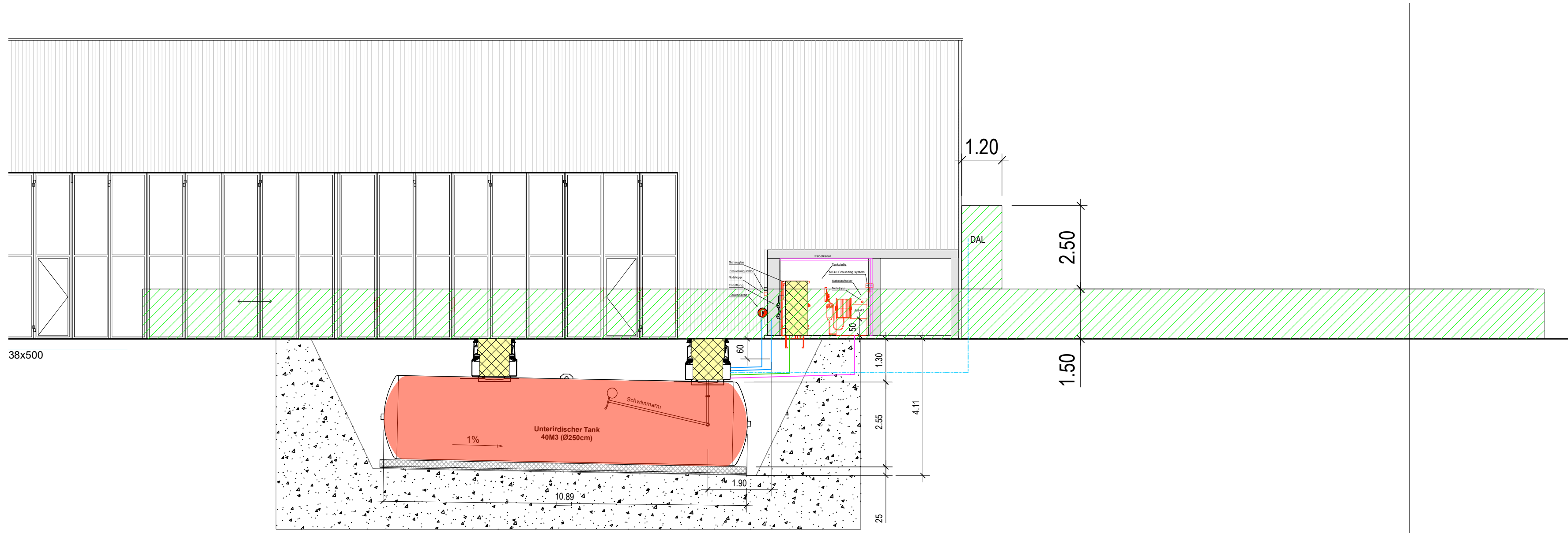
Längsschnitt Ech. 1/100
