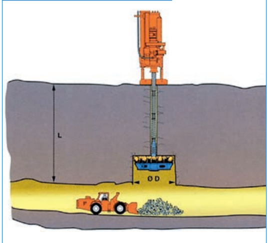
Schema raise boring Verfahren
